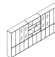
E99-2 W4364*D400*H2005(mm)
